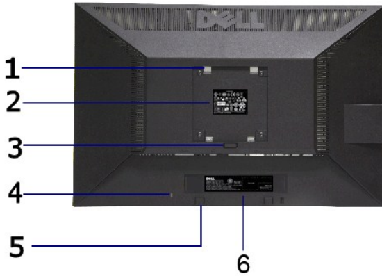
Tampilan Belakang
