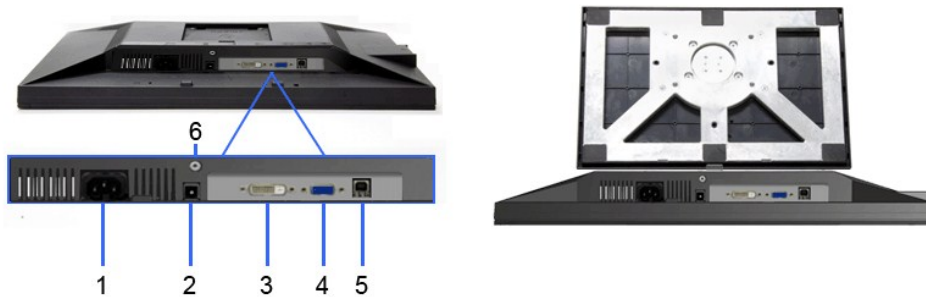
Tampilan Bawah
